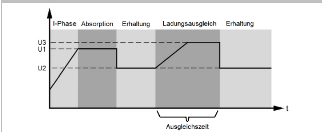
Abbildung. 2: Funktionsbeschreibung – Akkubank-Ladungsausgleichs-Funktion
