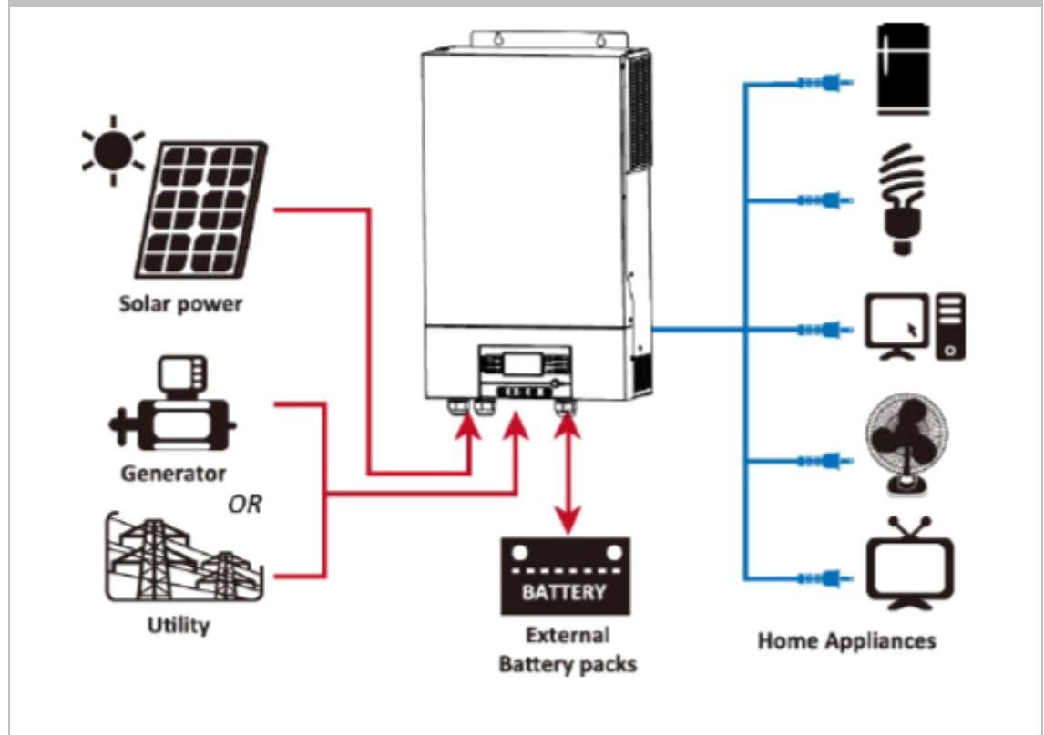
Abbildung. 3: Funktionsbeschreibung
