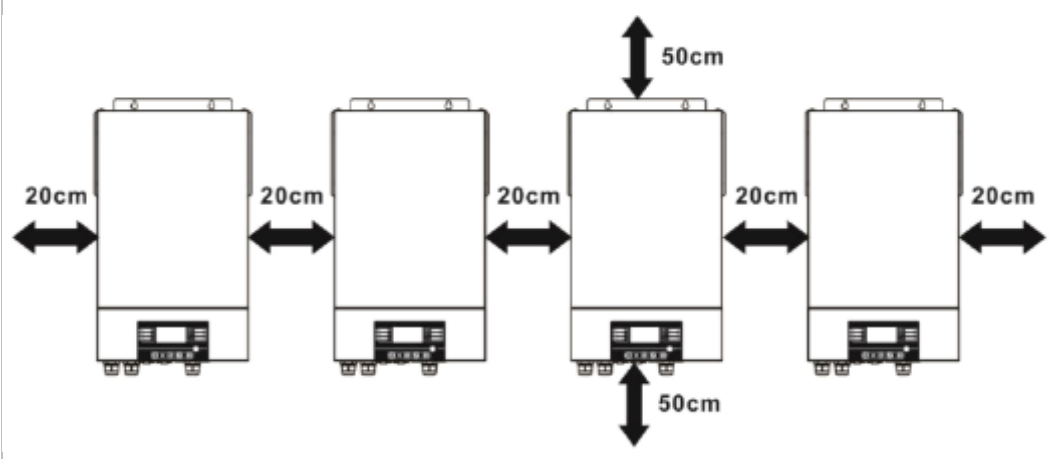
Abbildung. 1: Anschließen - Mehrere Geräte im Parallelbetrieb -
