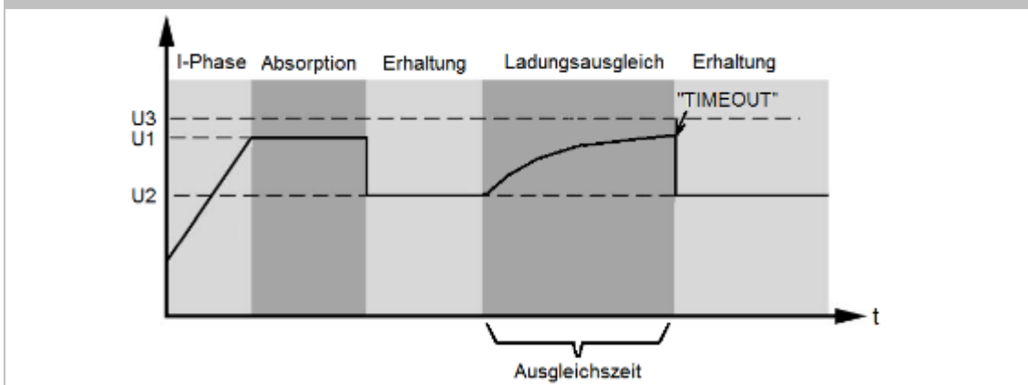
Abbildung. 3: Funktionsbeschreibung – Akkubank-Ladungsausgleichs-Funktion
