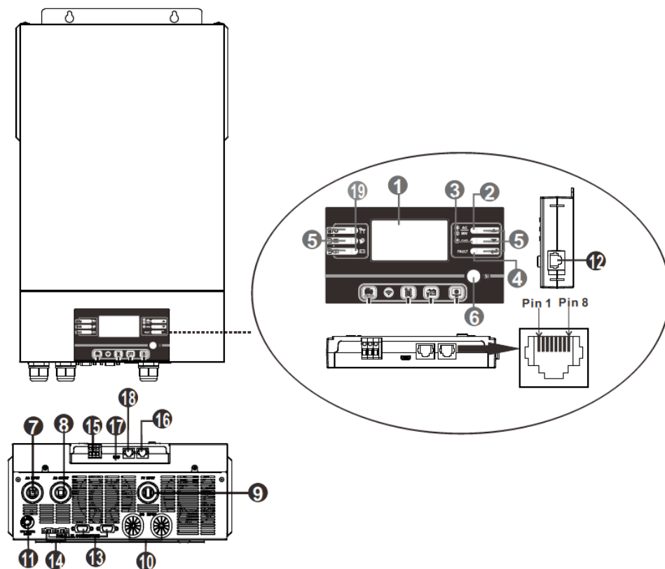
Abbildung. 2: Gerätebeschreibung
