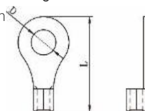
Ringkabelschuh:
